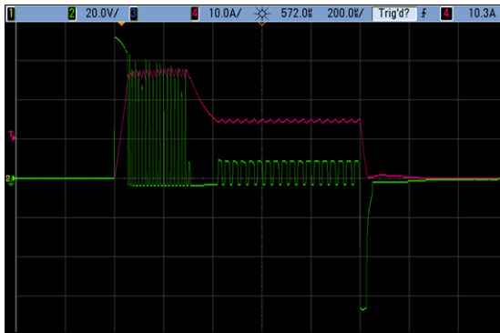
Figure 14. BackBoostTime = 0.100 ms
